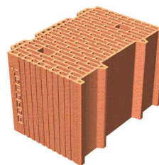
Blocco rettificato POROTON® denominato "IP35 SS DPE", dimensioni nominali 230 x 350 x 233 mm
