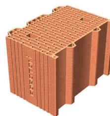
Blocco POROTON® denominato "P600 IT35 SS", dimensioni nominali 230 x 350 x 240 mm
