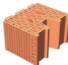
Blocco POROTON® denominato "P700 IP30", dimensioni nominali 240 x 300 x 190 mm
