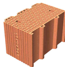
Blocco rettificato POROTON® denominato "P700 IP38 SS ECO DRY-PLAN", dimensioni nominali 230 x 380 x 233 mm
